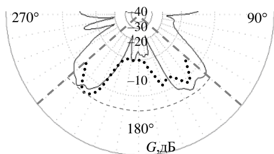
Рис. 4. Сравнение расчетной и измеренной диаграмм распределения ЭМП в горизонтальной плоскости для частоты 338 МГц (сплошная линия – расчетная диаграмма распределения ЭМП; прерывистая линия – измеренная диаграмма распределения ЭМП)
