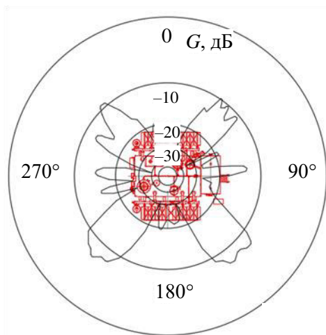
Рис. 3. Относительное распределение ЭМП автотрансформатора в горизонтальной плоскости в диапазоне частот 325...345 МГц
