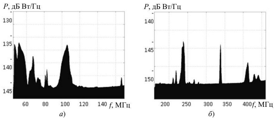
Рис. 2. Спектральные плотности мощности ЭМП АТ, измеренные с угла 210° в диапазонах частот, МГц: a – 45...170; б – 160...460
